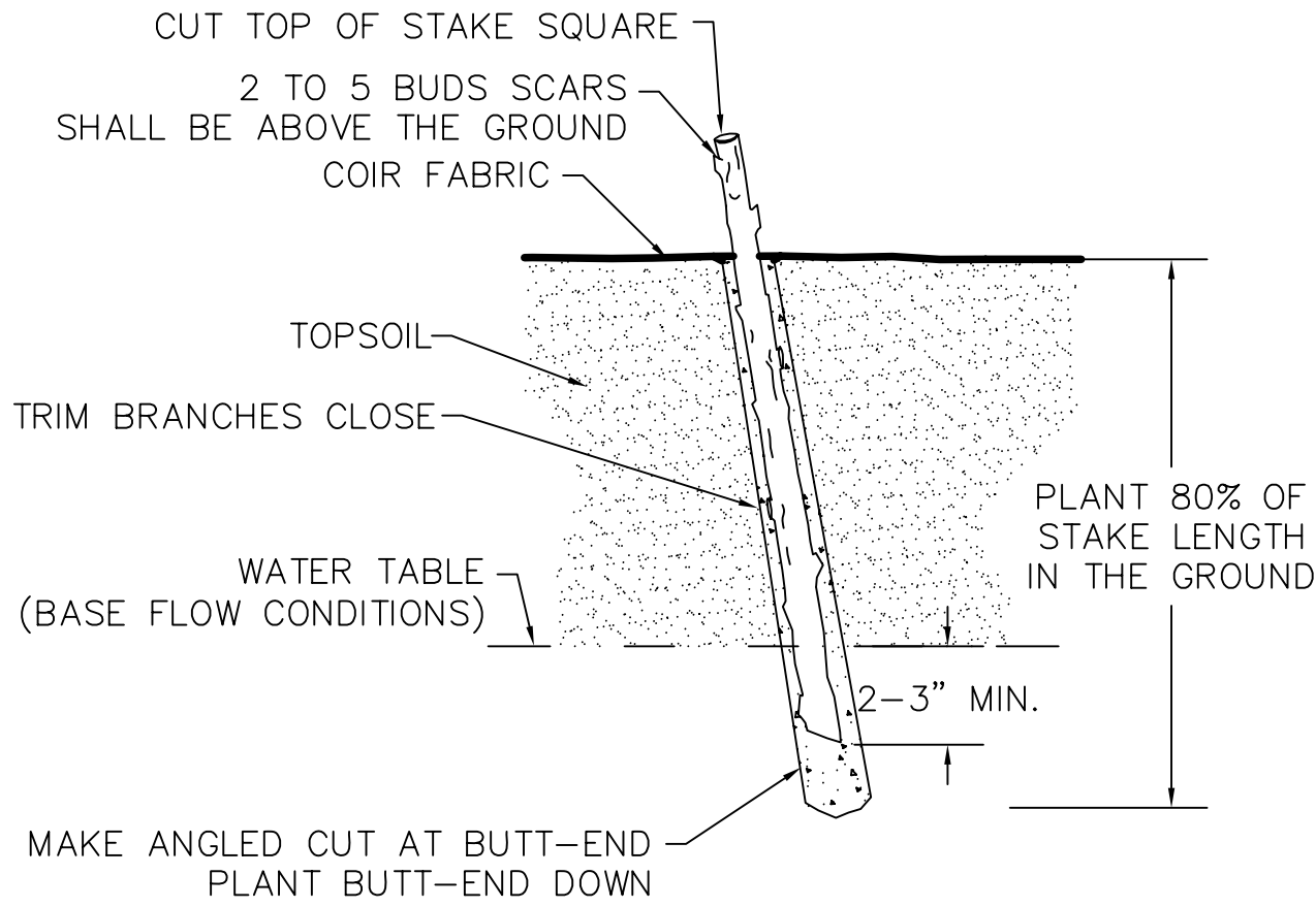
SECTION (TYP.)
